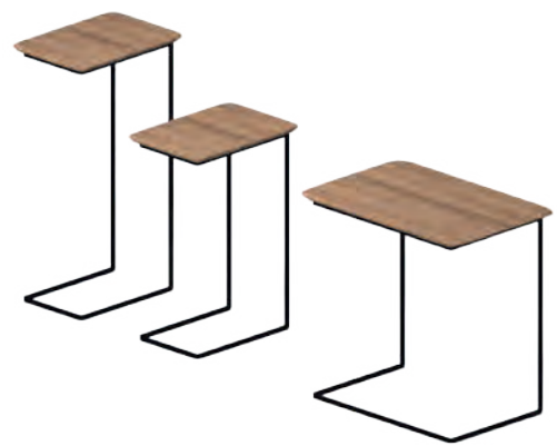
(COD. SELT0054) SERVETTO ALTO 25X35xh65 (COD. SELT0055) SERVETTO BASSO 25X35xh52 (COD. SELT0061) SERVETTO BASSO 55x35xh52
